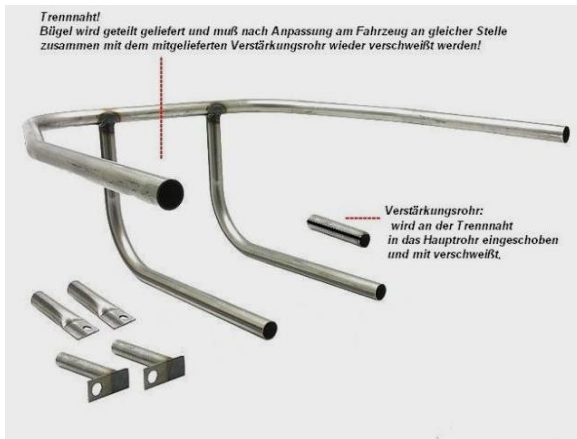
Motorschutzbügel „Universal“
