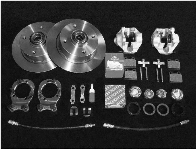
Umbausatz auf Scheibenbremsanlage
