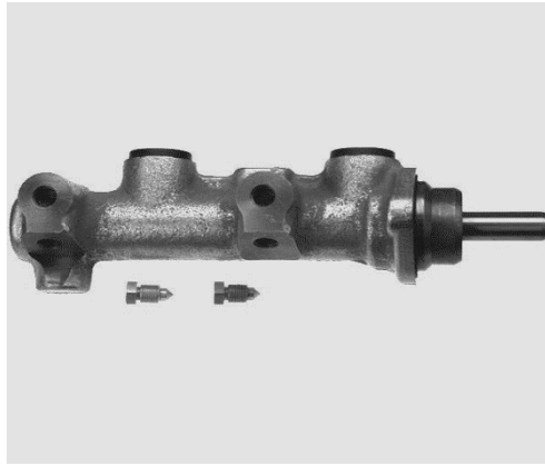
Spezial-Tandem-HBZ, 20,64mm
