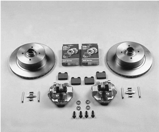
innenbelüftete Scheibenbremsanlage vorn
