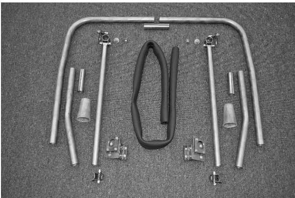
Überrollbügel-Kit
