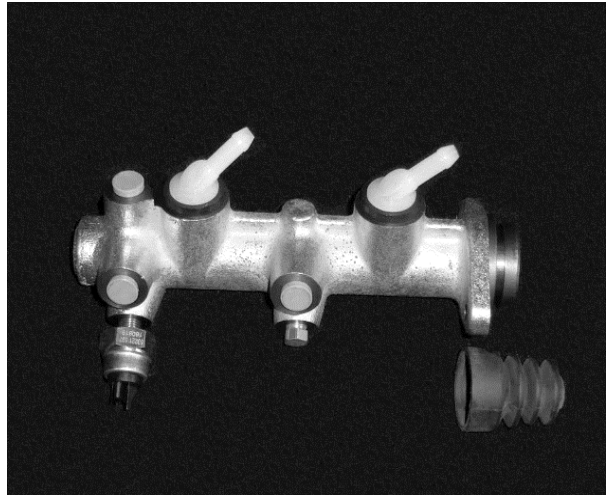
passender Tandem-Hauptbremszylinder dazu
