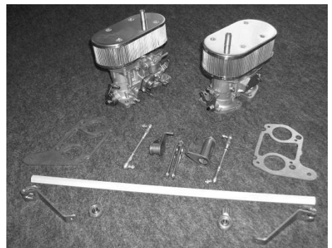
Weber 40IDF-Doppelvergaseranlage
